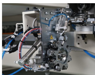
自动换梭装置 (选配) Automatic bobbin changer (Optional)
