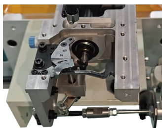
底面线自动剪线 Automatic Upper/Bobbin thread trimmer
